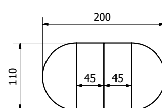
Stół rozkładany \phi 110 + 2 \times 45 cm
