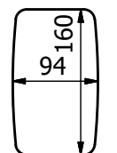
Stół spiek+szkło lub spiek+MDF
