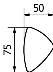
Ława spiek+MDF h = 42 lub h = 48
