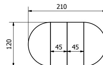
Stół rozkładany \phi 120 + 2 \times 45 cm
