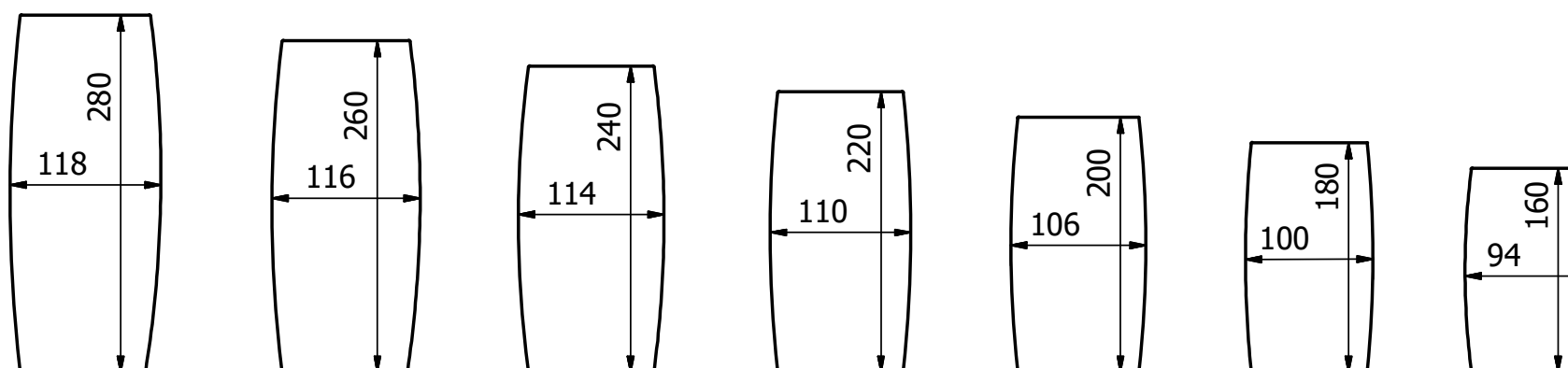
Stoły z blatem wykonanym z drewna orzecha amerykańskiego o wysokości 76cm.
